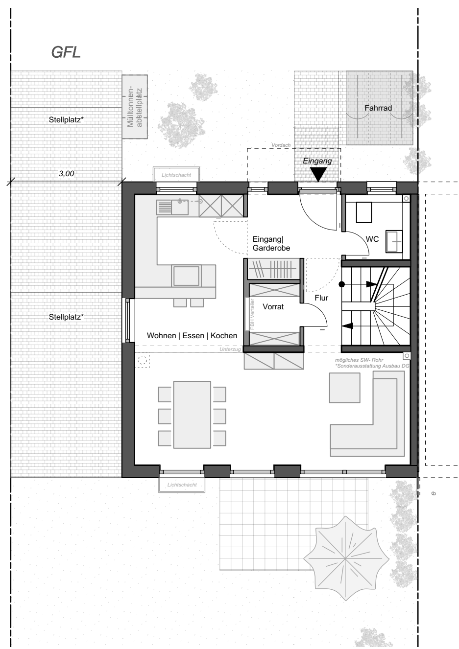
Erdgeschoss
