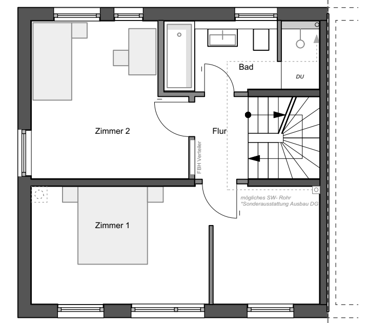
Obergeschoss
