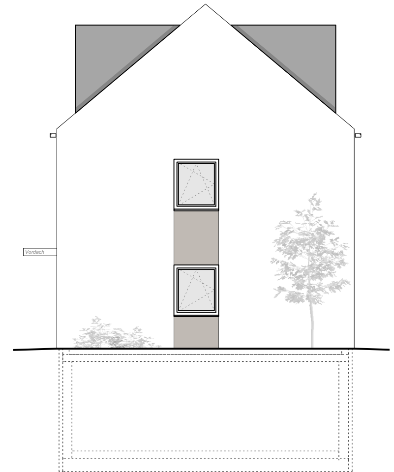
Ansicht West
