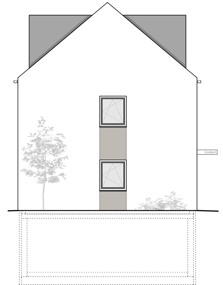
Ansicht Ost
