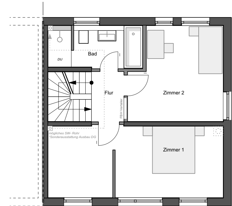
Obergeschoss
