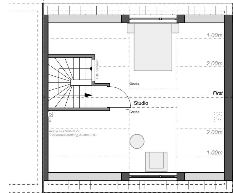
Dachgeschoss
