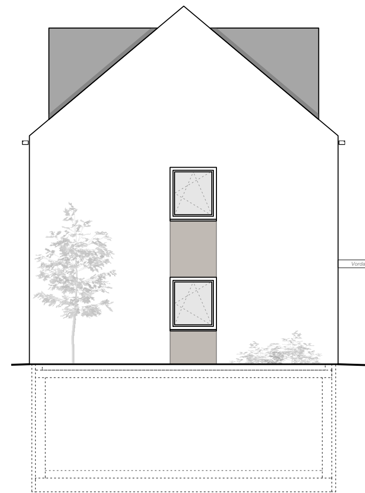
Ansicht Ost
