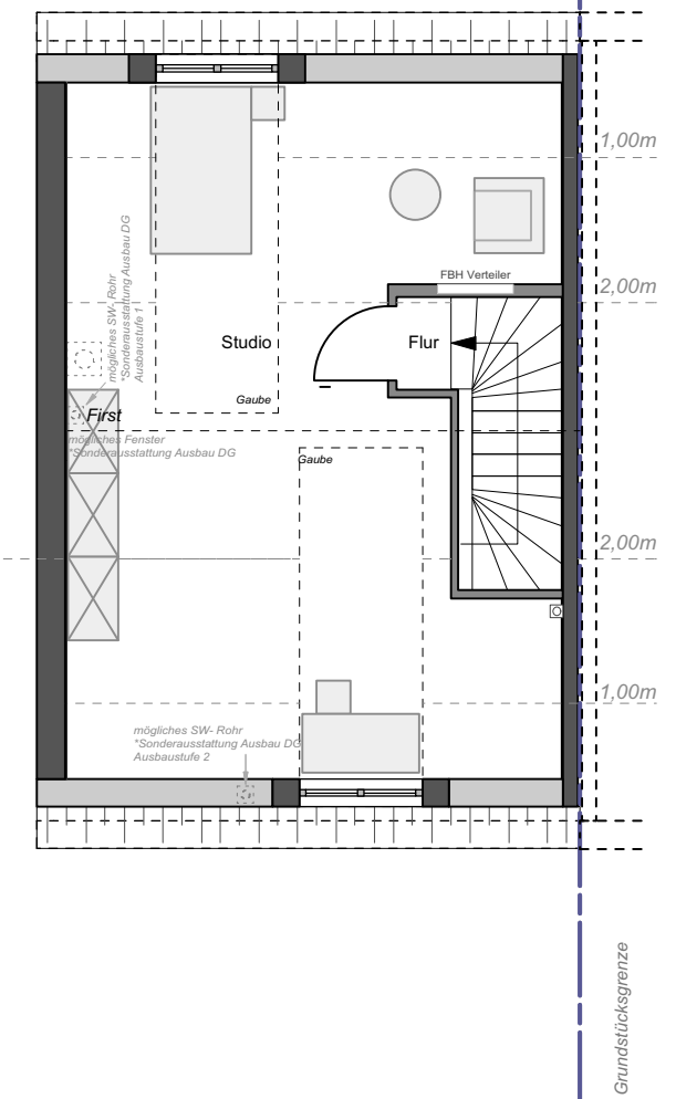
Dachgeschoss A 1.117d
