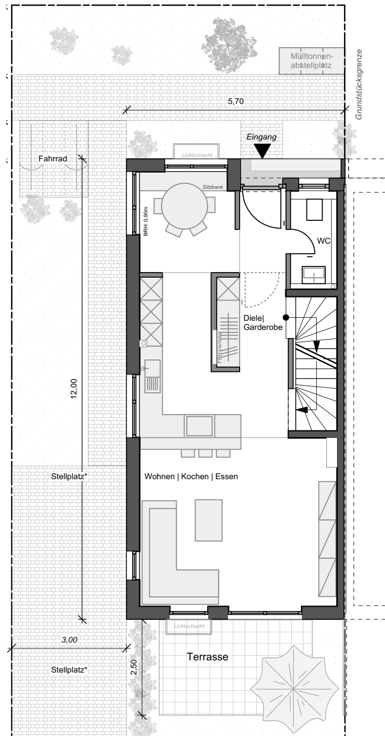
Erdgeschoss
