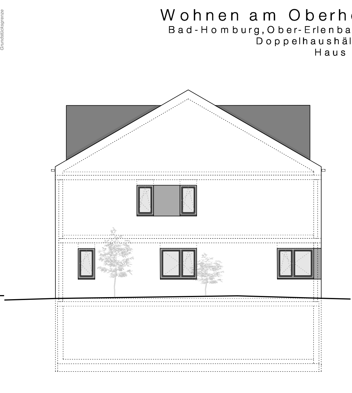
Ansicht Ost
